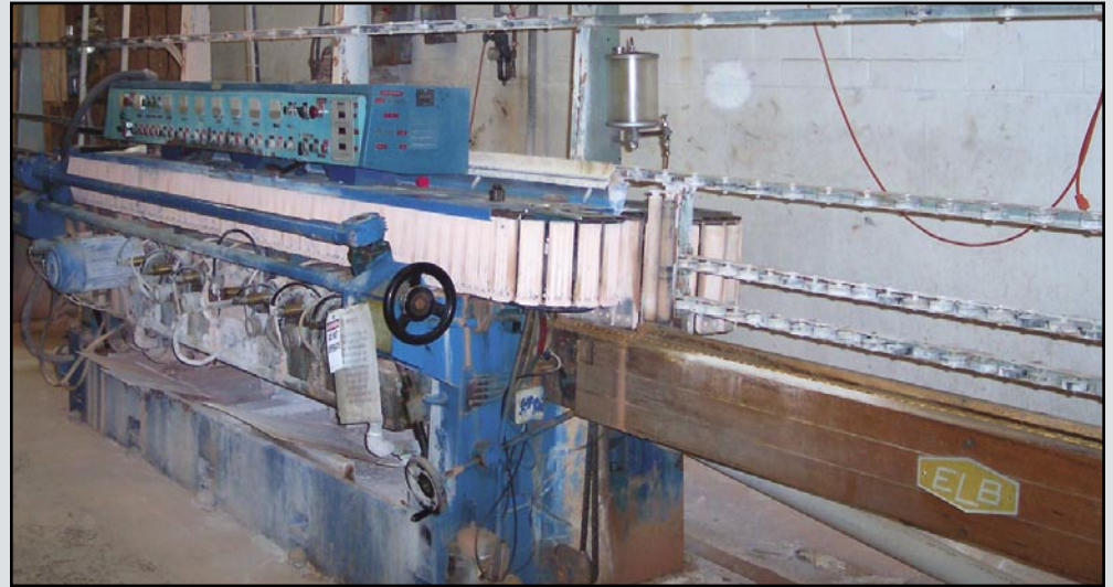
BEVELING MACHINE
